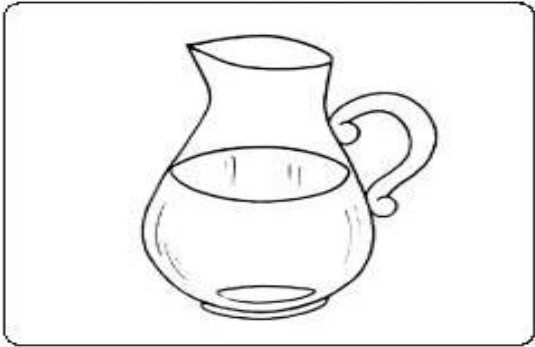
Estado líquido
