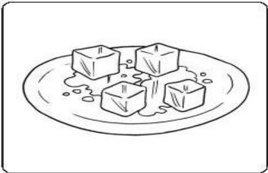
Estado sólido
