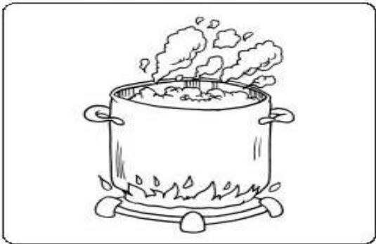
Estado gaseoso
